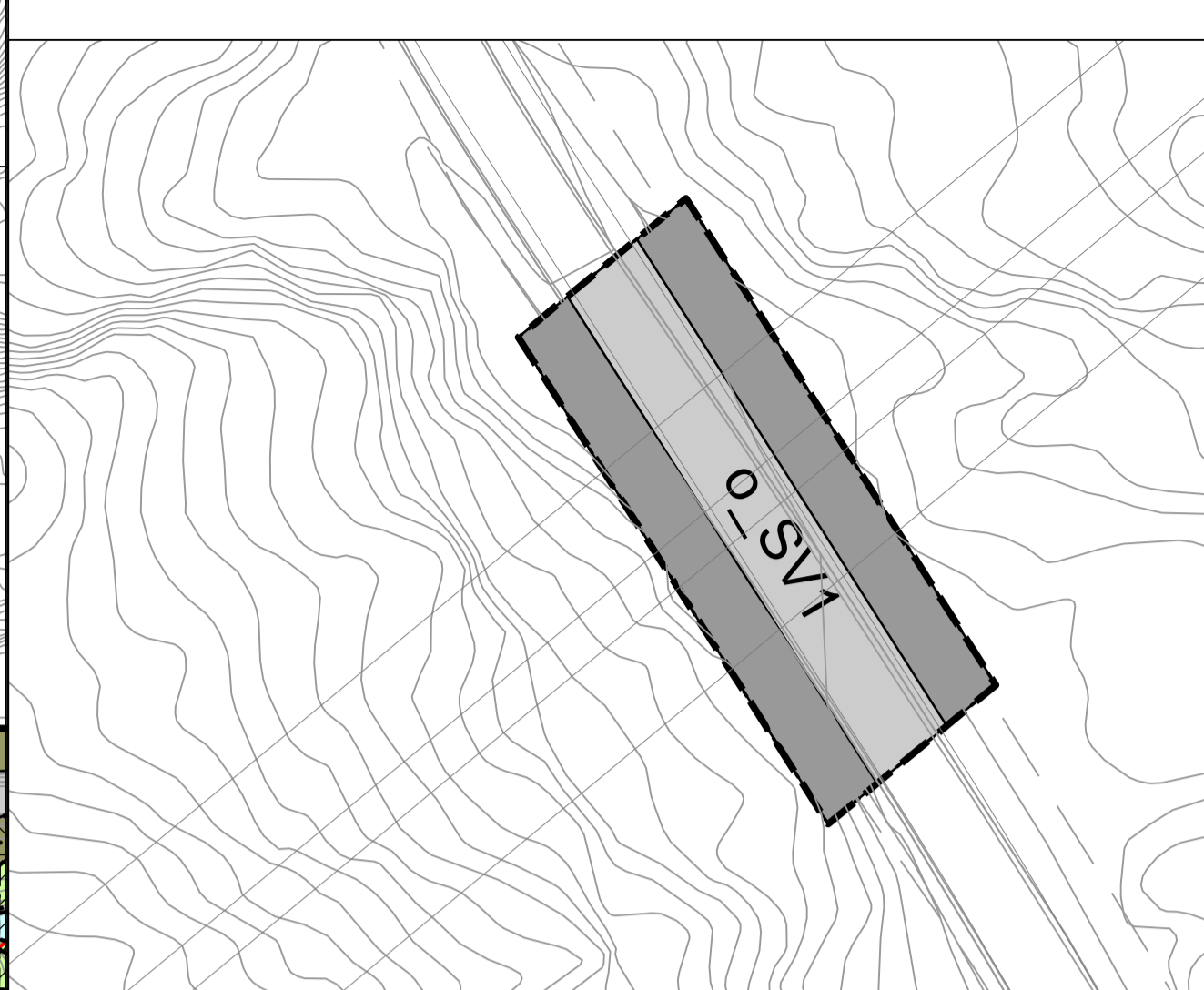
Vertikalnivå 3 - Over grunnen (bru) M = 1:500
