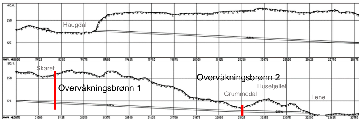
Figur 33: Lengdeprofil langs Eikeråsheiatunnelen (Fra tegning V3014 i vedlegg 1). Røde streker viser ca. plassering av overvåkningsbrønner
