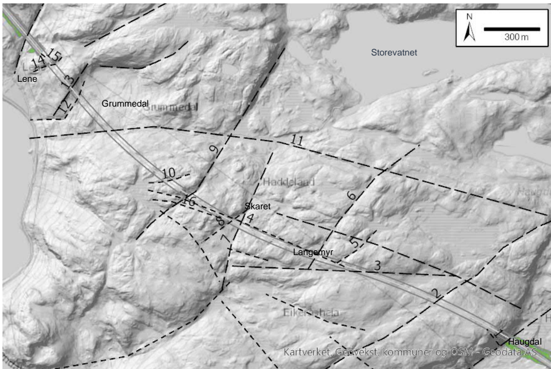
Figur 14: Kartlagte lineamenter i området over Eikeråsheiatunnelen. Hvert enkelt lineament er nummerert.
