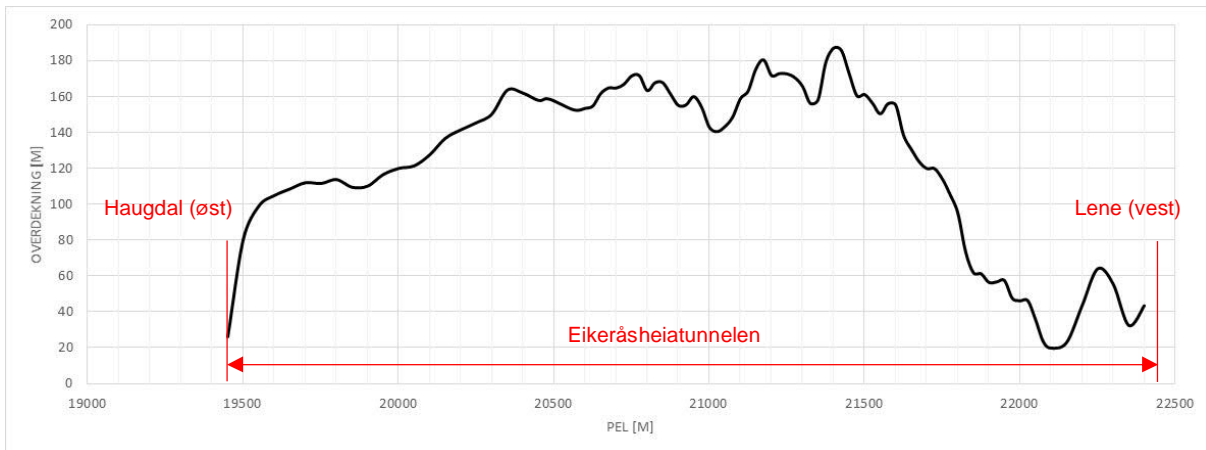
Figur 19: Diagram som viser vertikal bergoverdekning for senterlinjen mellom tunnellopene mot pelnummer.
