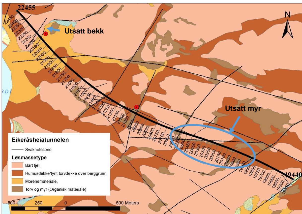
Figur 34: Kart som illustrerer løsmassen og utsatte naturtyper som må hensyntas i vurderingen av innlekkasjekrav for Skreihei-tunnelen. Store og små svakhetssoner krysser tunnelen og markert med svarte små streker (Løsmassedekke er tatt fra NGU).
