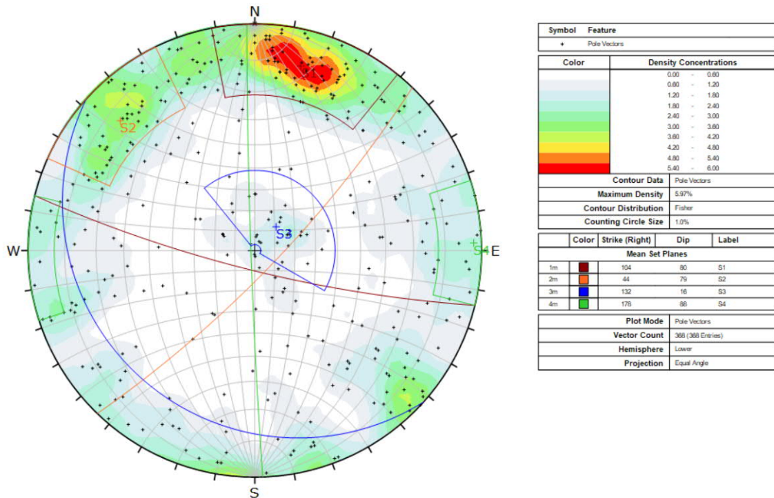
Figur 13: Konturplott av alle sprekemålingene over Eikeråsheiatunnelen med definerte sprekkesett.
