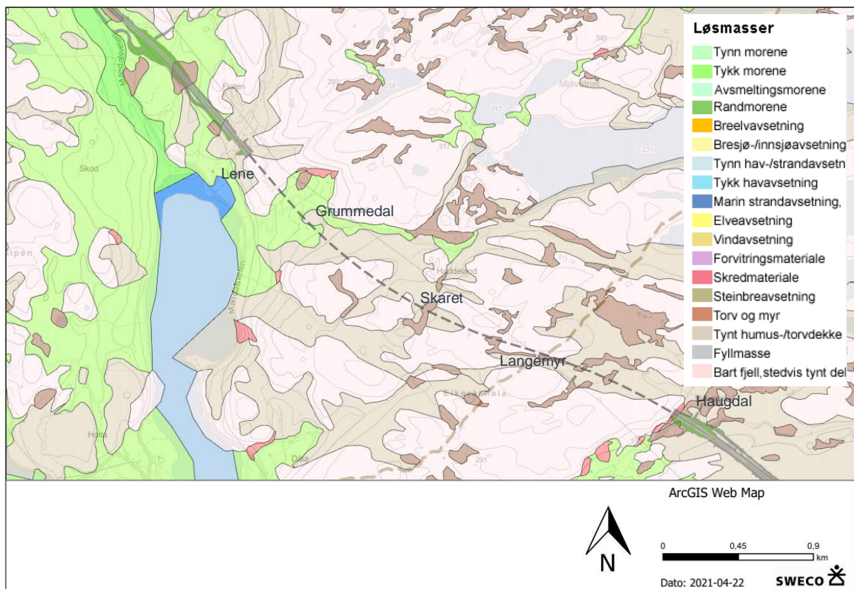
Figur 9: Kvartærgeologisk kart [7]. Stort sett bart berg eller tynt humus-/torvdekke over tunnel (stiplet).
